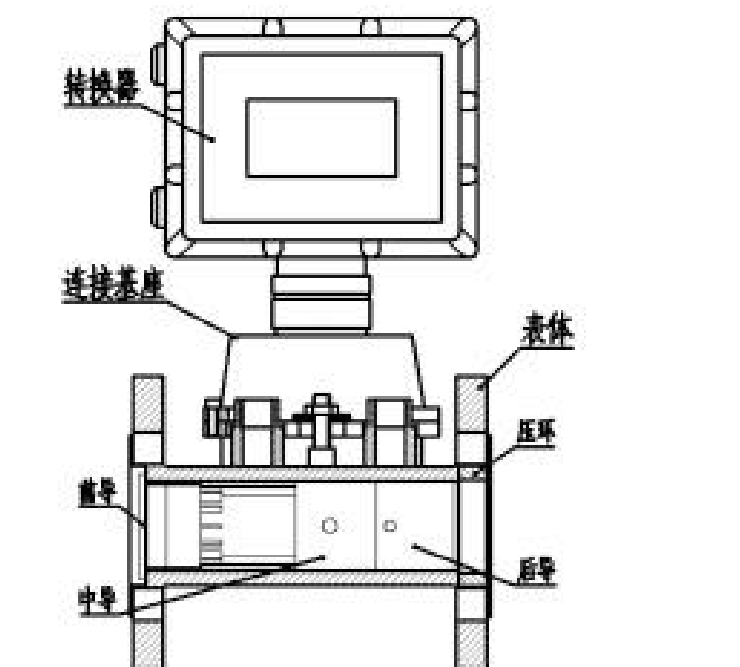
图 1-1 法兰连接型涡轮流量计结构图
