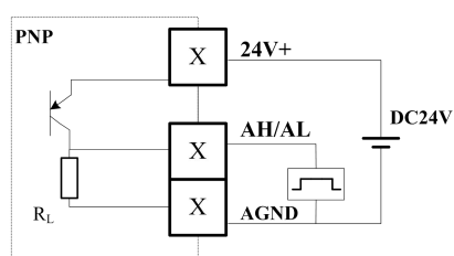
图 5-7 三线制供电报警输出接线图
