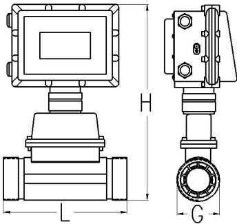
图 4-1 螺纹连接示意图
